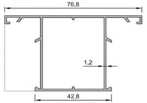
No : 1604 Geniş Orta Kayıt 0,760 kg/m
