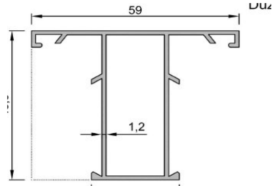
No : 1601 Dar Orta Kayıt 0,645 kg/m
