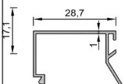
No : 1507 Tek Cam Çıtası 0,210 kg/m
