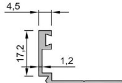
No : 1510 Jaluzi Cam Çıtası 0,210 kg/m
