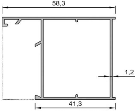
No : 1607 Geniş Kasa 0,660 kg/m
