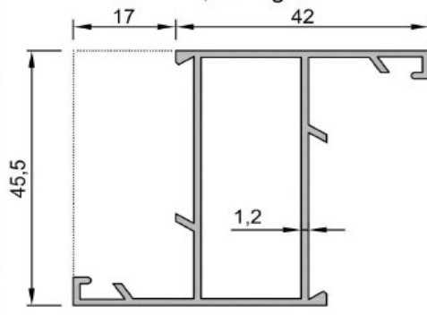
No : 1602 Dar Kanat 0,645 kg/m
