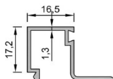
No : 1508 Isı Cam Çıtası 0,260 kg/m
