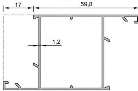
No : 1605 Geniş Kanat 0,760 kg/m
