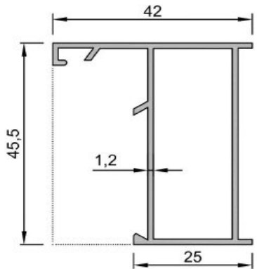
No : 1603 Dar Kasa 0,545 kg/m
