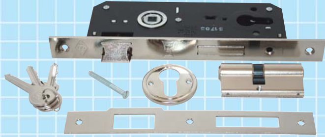
A 3004 Geniş dilli kilit Çift turlu 35 mm
