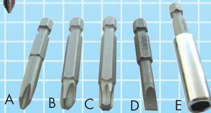
A 201 Vidalama ucu
