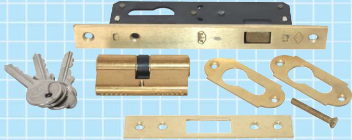
A 3006 Sürme kilit barelli
