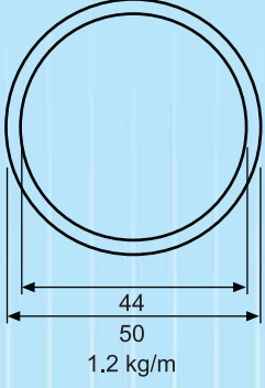
Küpeşte 50'lik boru
