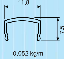
Küpeşte dikme kapağı
