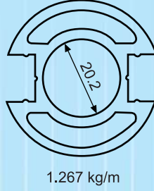
Küpeşte dikme profili
