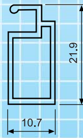
0.200 kg/m Küçük sineklik profili
