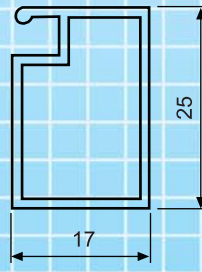
0.260 kg/m Büyük sineklik profili
