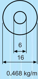
Küpeşte 16'lik boru
