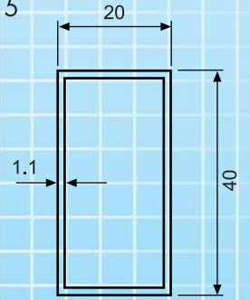
0.375 kg/m 40X20 kutu sineklik profili
